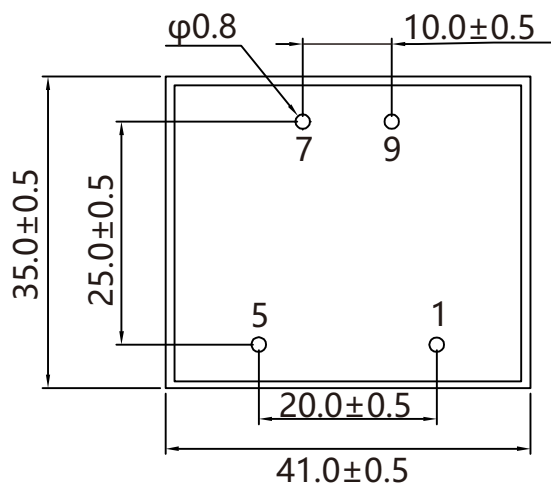
底部视图
