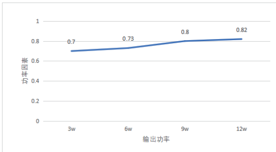
功率因数VS输出功率
