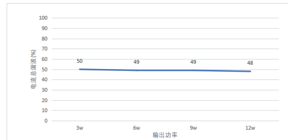
电流总谐波VS输出功率
